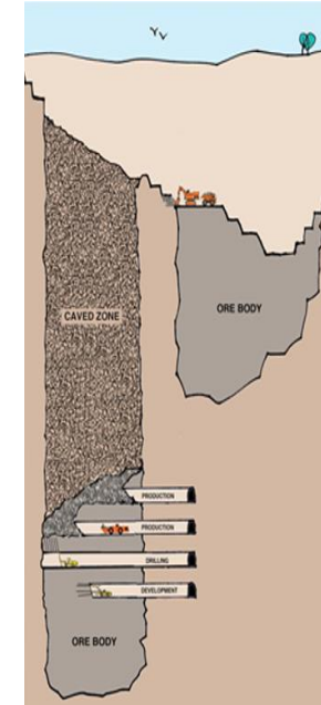
Sublevel Caving
